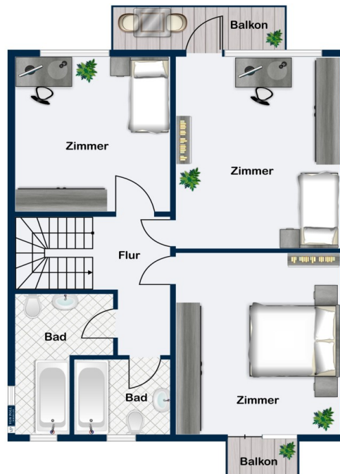
1. Obergeschoss
