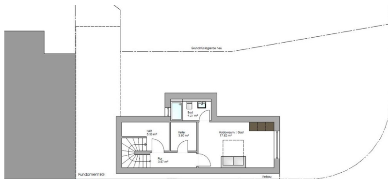
KELLERGESCHOSS EFH WOHFÄCHE ca. 25,44m² Nutzfläche ca. 17,91m²
