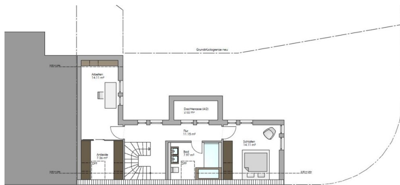
DACHGESCHOSS EFH WOHFÄCHE ca. 54,71m²
