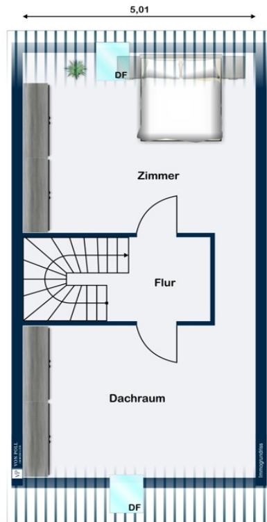
Dachgeschoss
