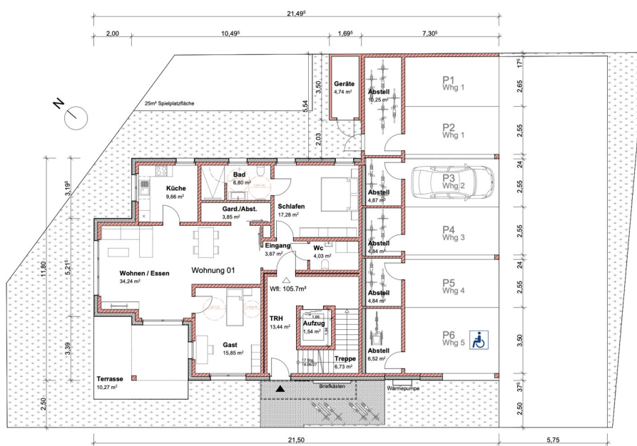
GRUNDRISS EG
