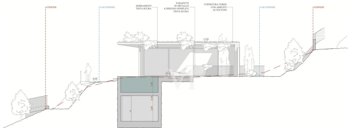
SEZIONE D 1:100
