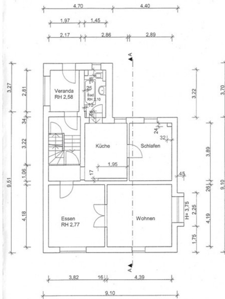
Grundriss Erdgeschoss
