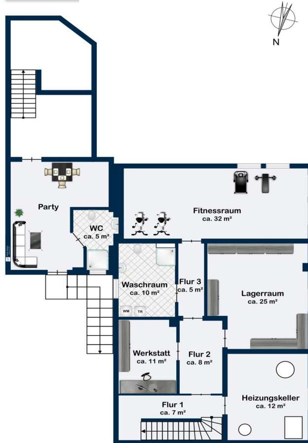
Untergeschoss
