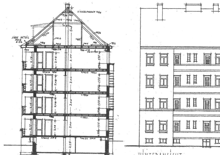
Schnittzeichnung
