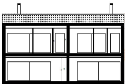
Sección A-A'.
