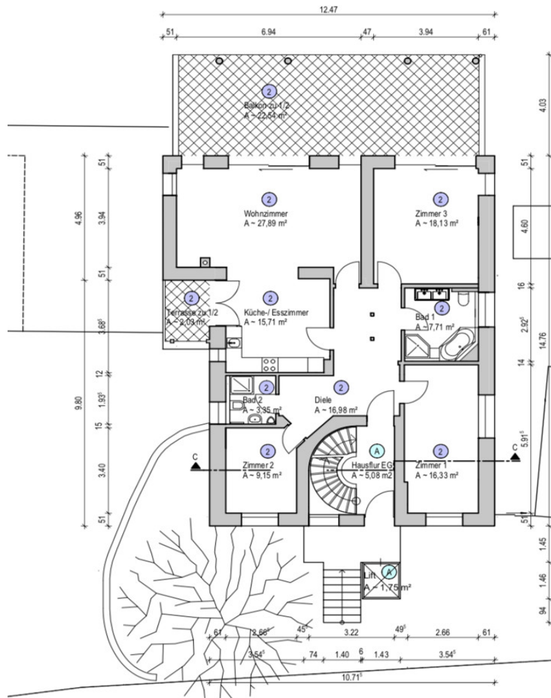
Grundriss Erdgeschoss
