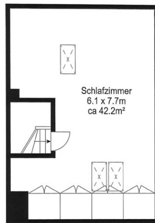
Dachgeschoss
