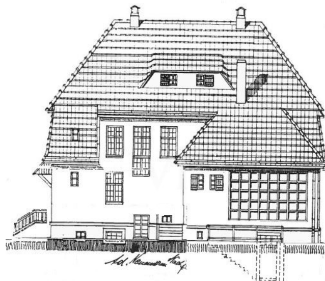
(Nord) Hinter-Ansicht.
