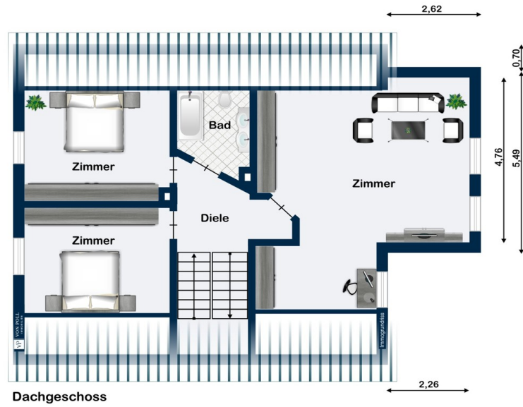
Dachgeschoss
