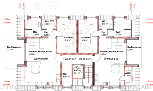
GRUNDRISS DG
