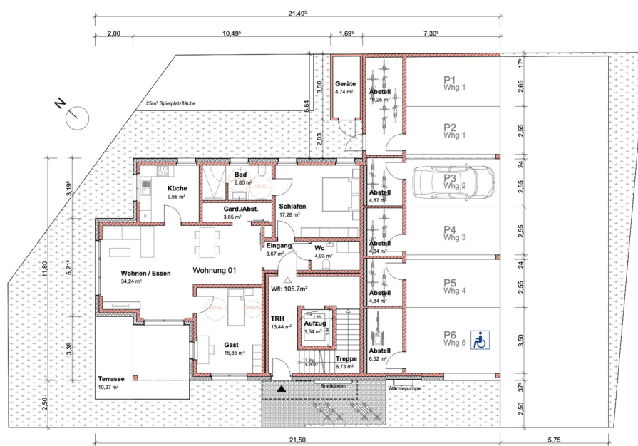
GRUNDRISS EG
