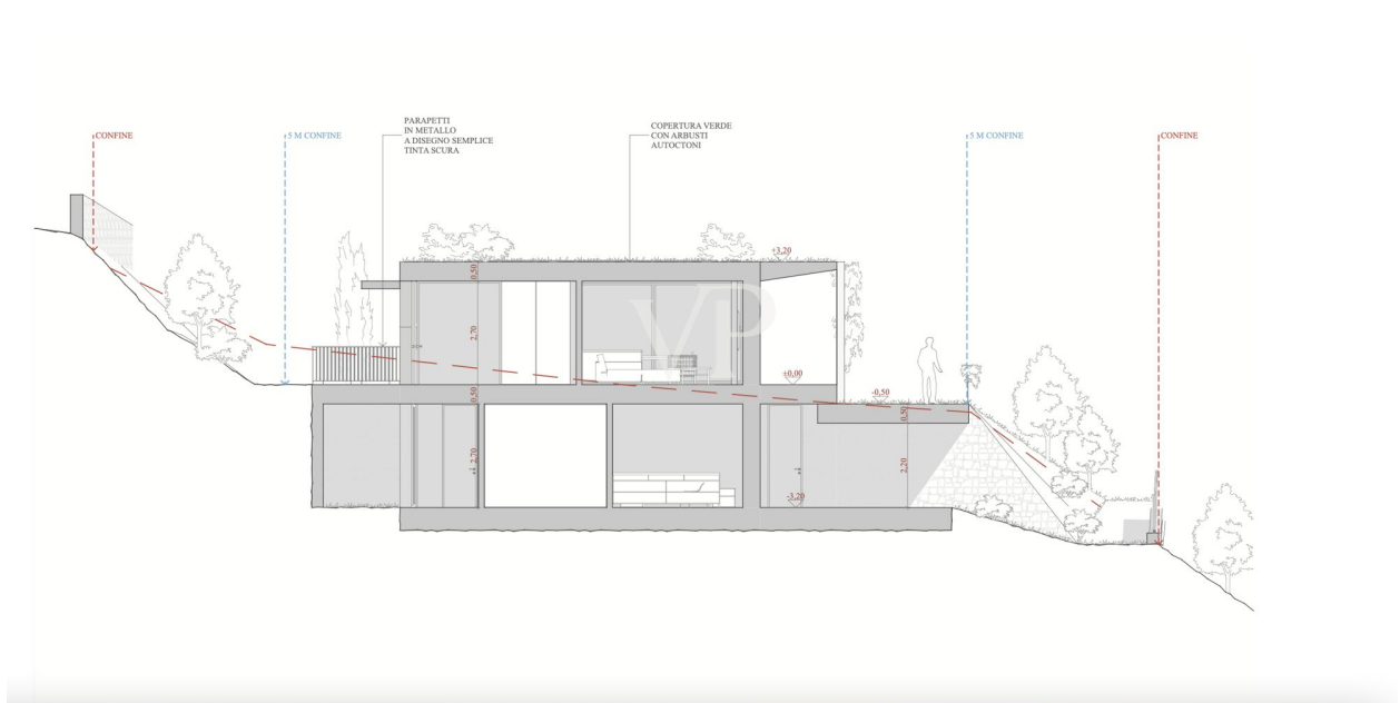
SEZIONE B 1:100
