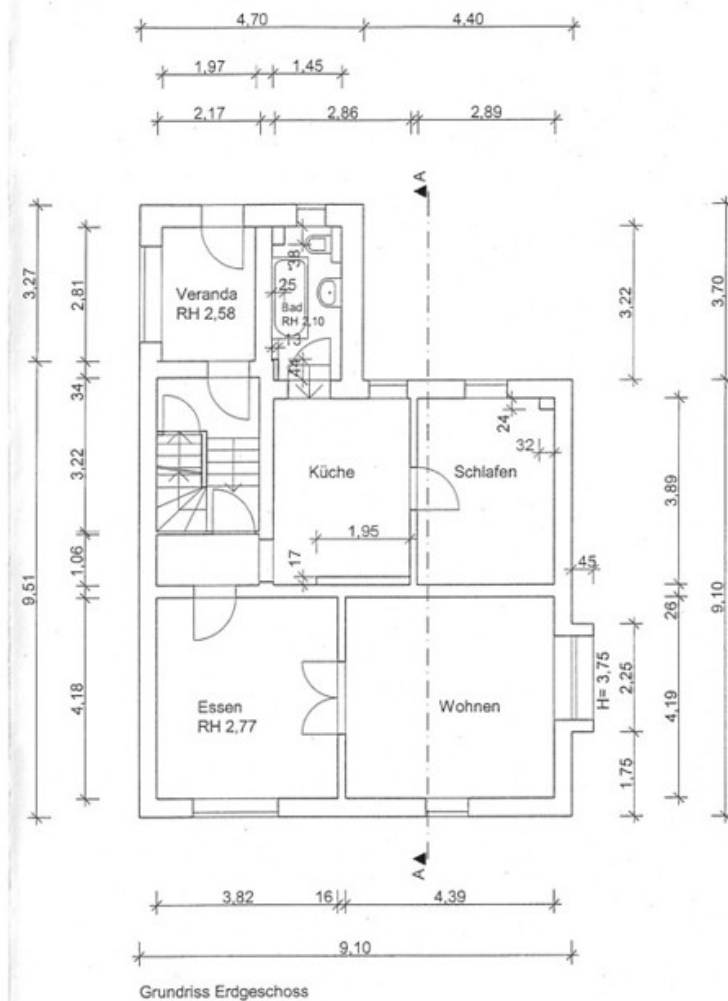
Grundriss Erdgeschoss
