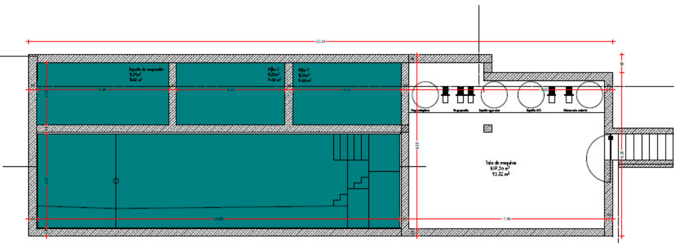
Representación plano de planta del primer nivel
