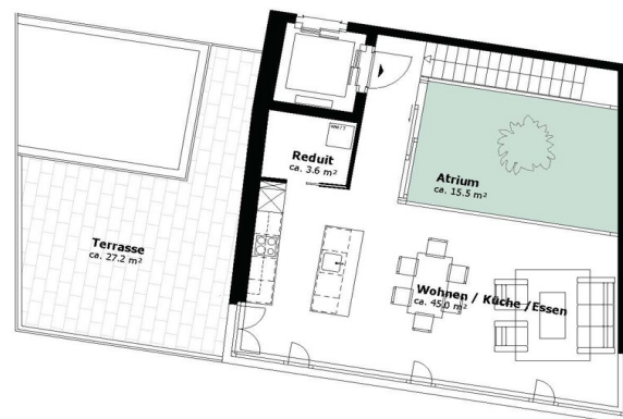
Dachgeschoss
