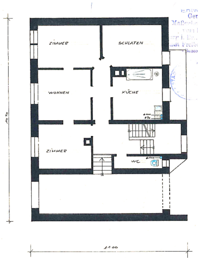
Erdgeschoss Vorderhaus
