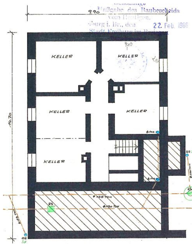
Kellergeschoss Vorderhaus
