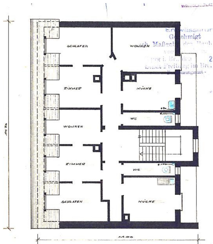
Vorderhaus Ober- /Dachgeschoss
