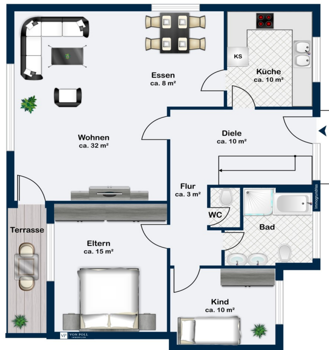
Erdgeschoss
