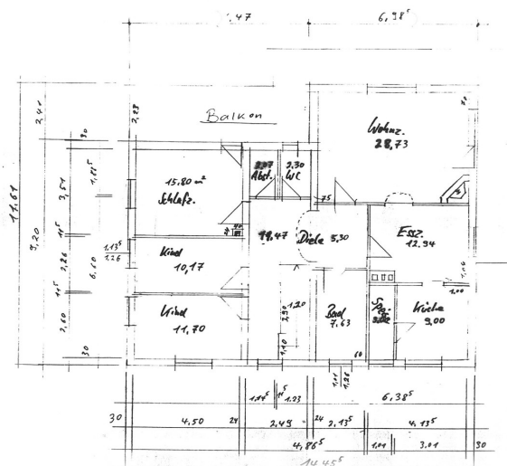
Grundriss Obergeschoss
